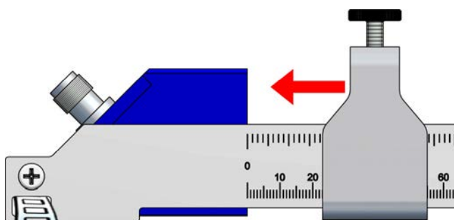
Fig. 4. Guía de posicionamiento y abrazadera de fijación DN80 ... DN350
