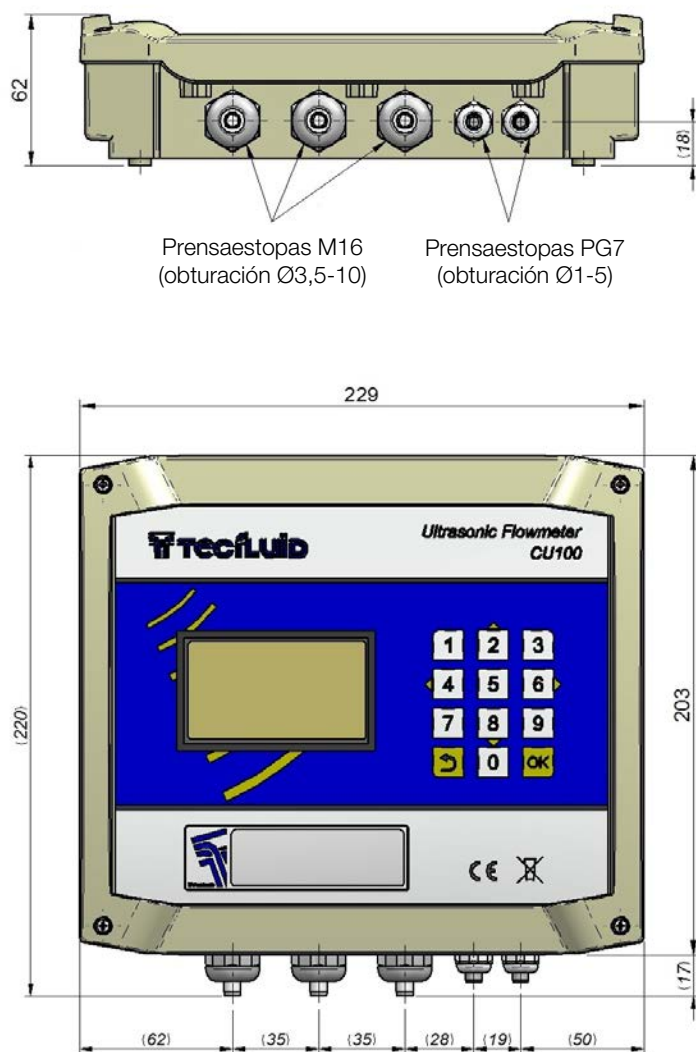
Fig. 7. Convertidor CU100
