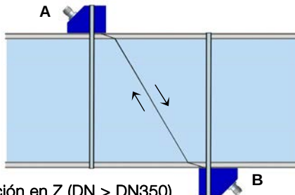
Fig. 2. Instalación en Z ( DN > DN350 )
