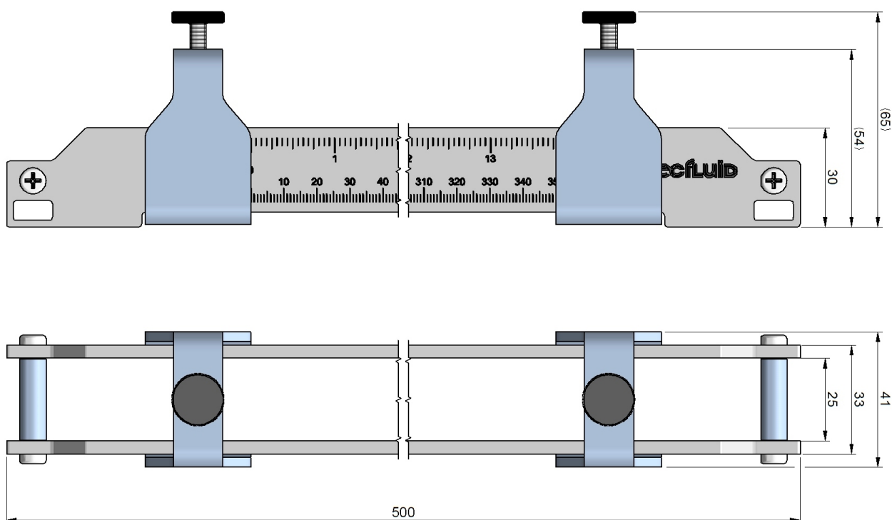
Fig. 8. Guía de posicionamiento (DN80 ... DN350)
