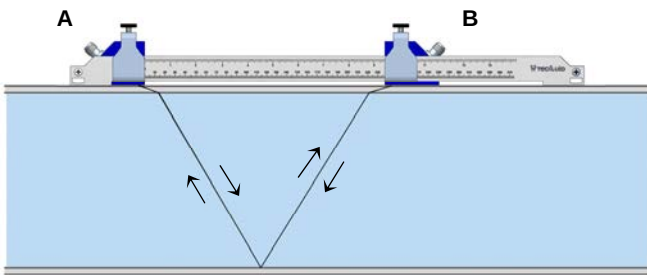
Fig. 1. Instalación en V ( DN \leq DN350 )
